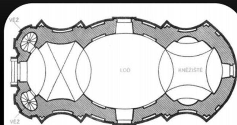
KŘIVKAMI TVOŘENÝ PŮDORYS VRCHOLNĚ BAROKNÍHO KOSTELA
