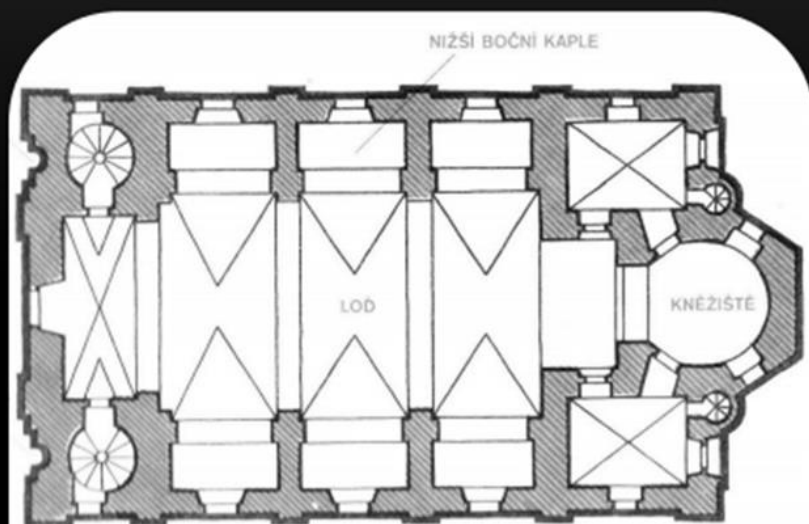
STROHÝ PRAVOÚHLÝ PŮDORYS RANĚ BAROKNÍHO KOSTELA
